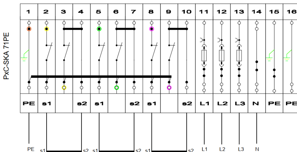
Schemat wewnętrzny listwy PxC-SKA 71PE
