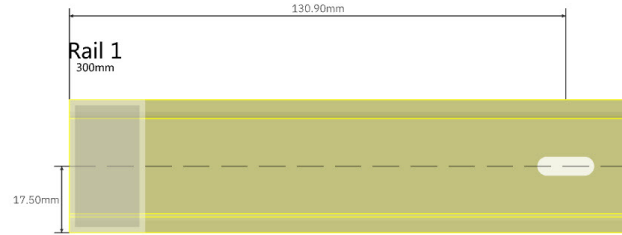
Şekil 6 Boyutsal bilgiler
