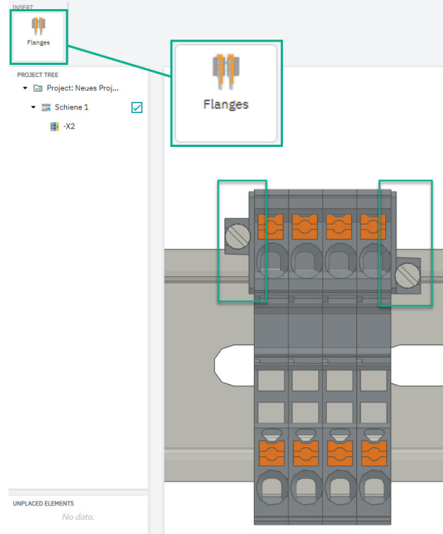
Şekil 9 Flanşlar
