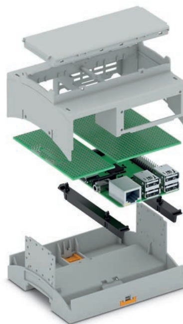
基本セット (Raspberry Piは含みません) RPI-BC 107,6 DEV-KIT KMGY (写真の基板はオプション)
