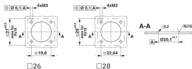
推奨穴あけ加工図
