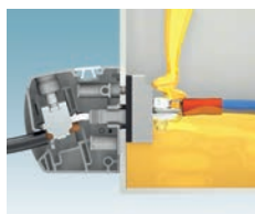
② ポッティング用 例) PW 4-POT... パネル内側 a. タブ端子、b. はんだ付け、 またはc. ねじ接続
