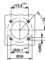
推奨穴あけ加工図 タイプ：2S
