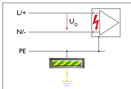
Fig. 4: Normal-mode voltage
