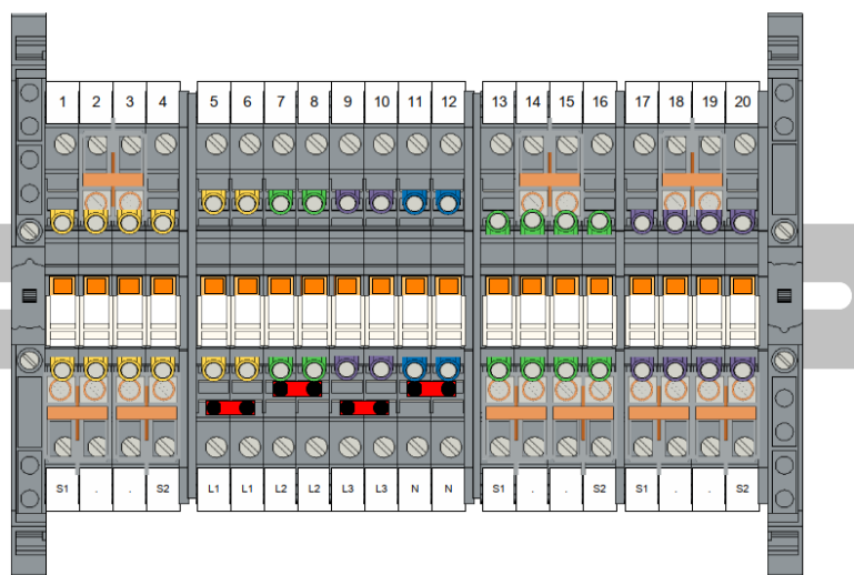
Złączka rozłączalna UTME 6
