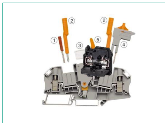
Akcesoria do złączki UTME 6
