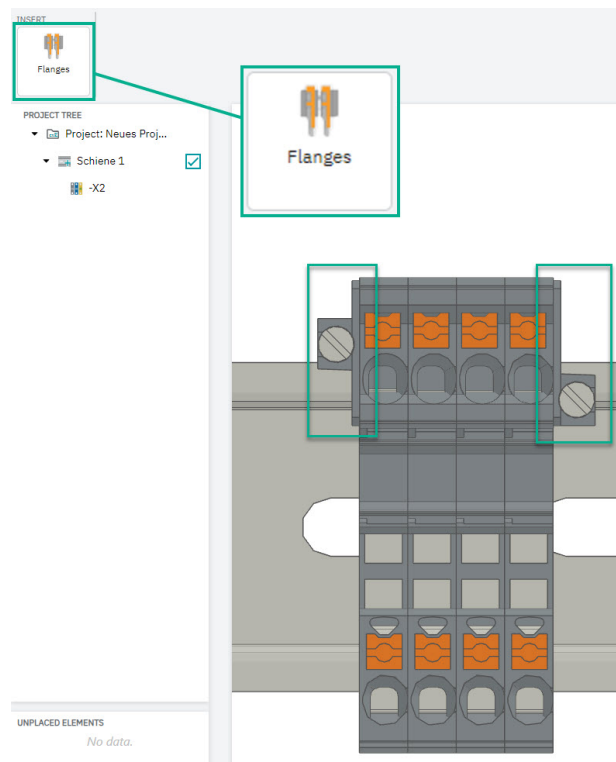
Ilustr. 9 Kołnierze
