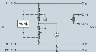
Innenschaltbild eines T3-Ableiters mit integrierter Vorsicherung
