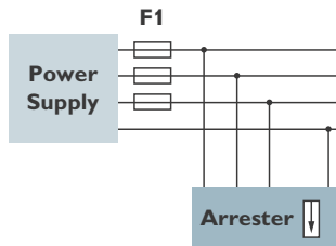
Installation direkt hinter der Anlagenvorsicherung
