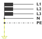
TN-S-System, 3-phasig
