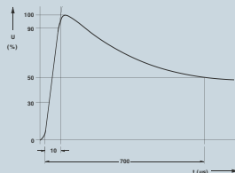
10/700 Stoßspannungsimpuls nach ITU-TK44
