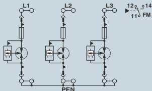
Innenschaltbild eines T1-Ableiters mit integrierter Versicherung
