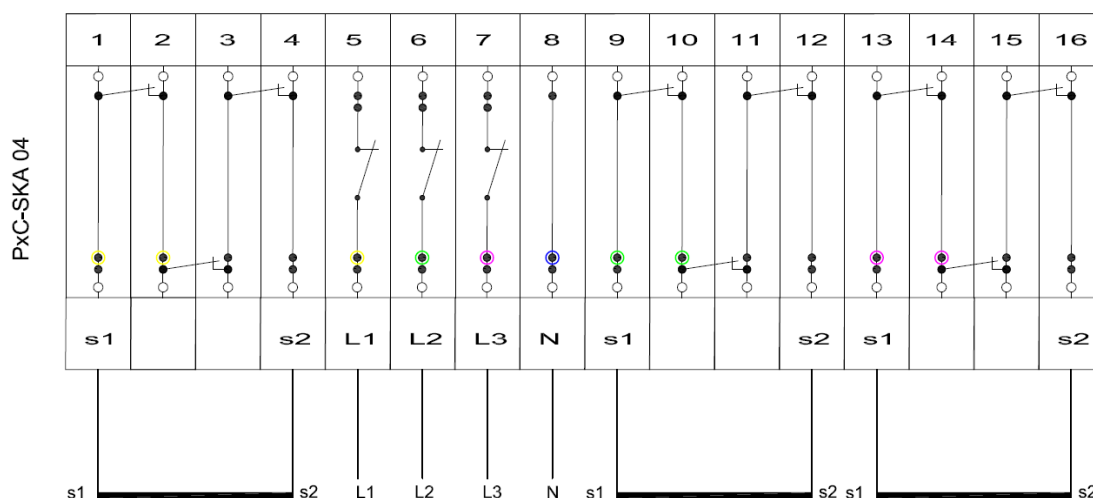
Schemat wewnętrzny listwy PxC-SKA 04
