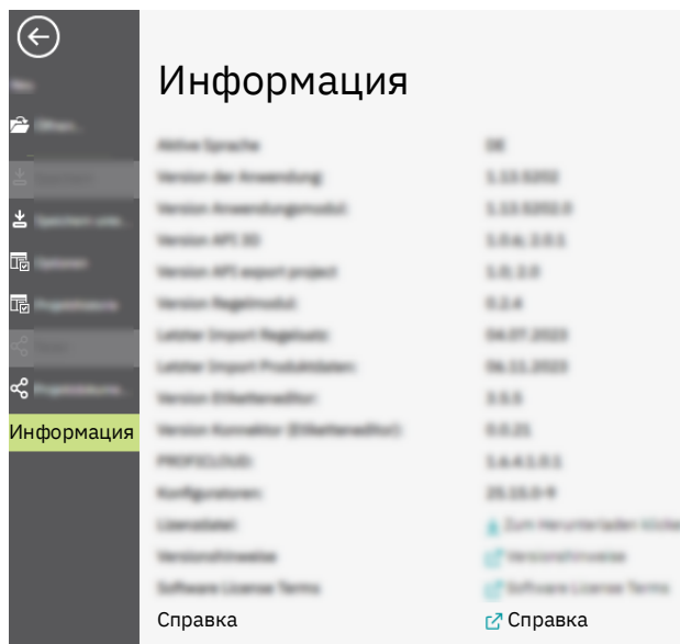
Рис. 1 Интерактивная справка
