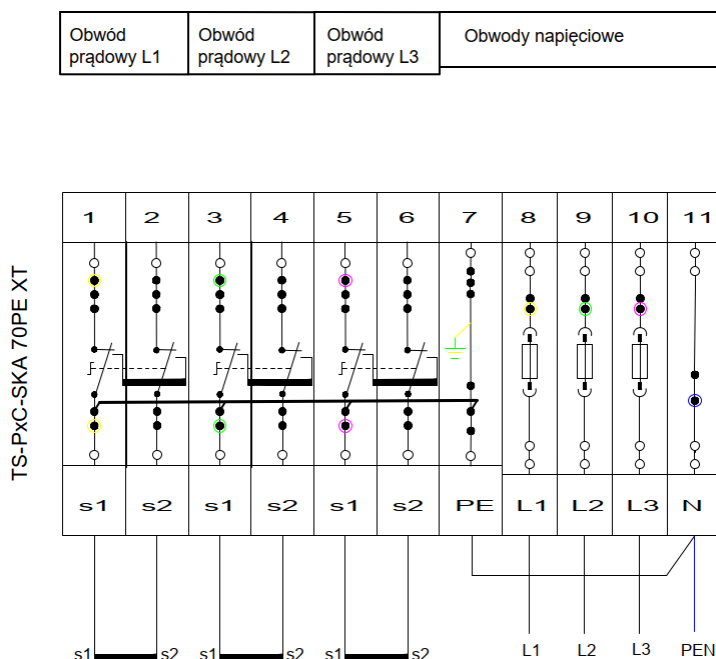
Schemat wewnętrzny listwy TS-PxC-SKA 70PE XT
