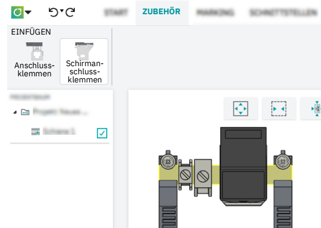
Bild 3 Neutralleiter-Sammelschiene
