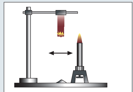
UL 94に準拠した試験治具
