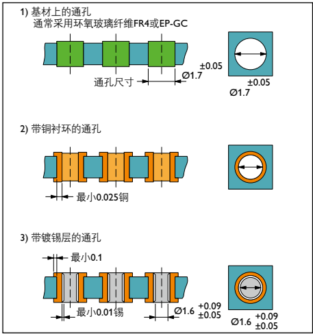
适配双排SDDC 1,5的通孔内径 (单位：mm)
