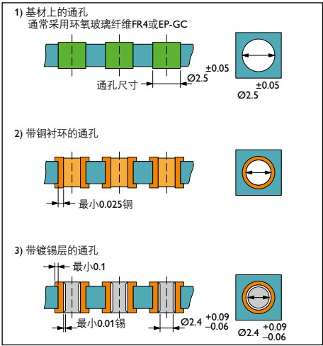
适配单排SDC 2,5的通孔内径 (单位：mm)
