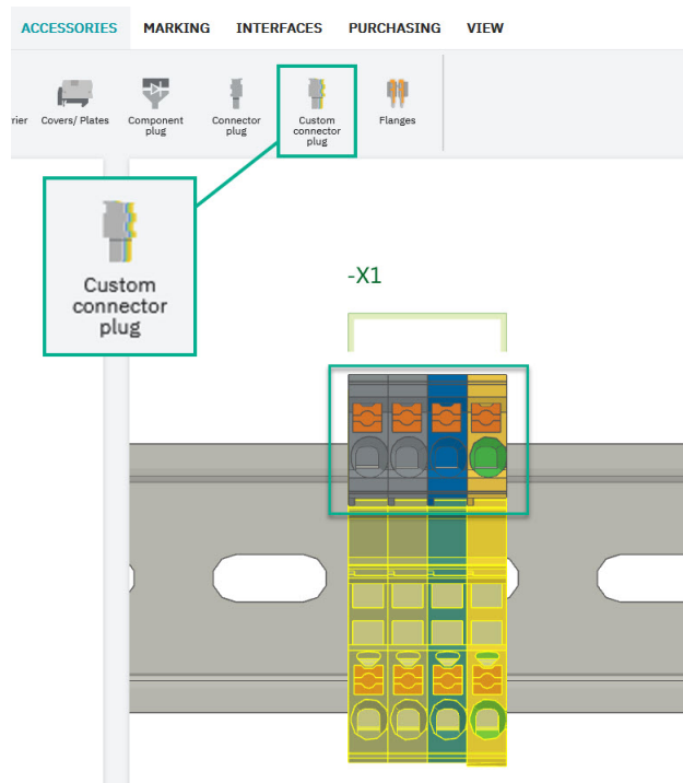
Figura 8 Conector personalizado
