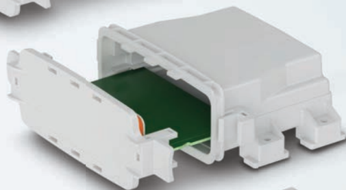
プリント基板のさまざま な厚さに対応する締め具
