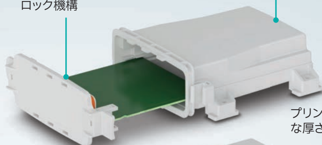
プリント基板の ロック機構
