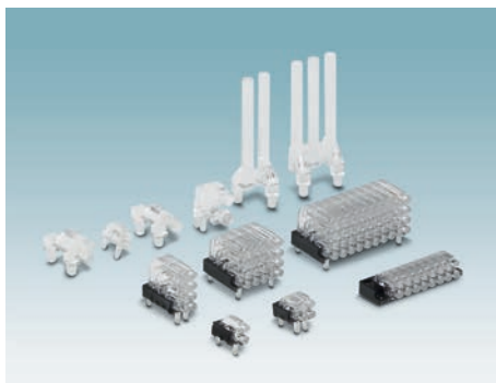
状態表示用に丸型または長方形配列の水平型および垂直型の導光パイプ
