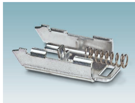
金属製と樹脂製のベースラッチ
