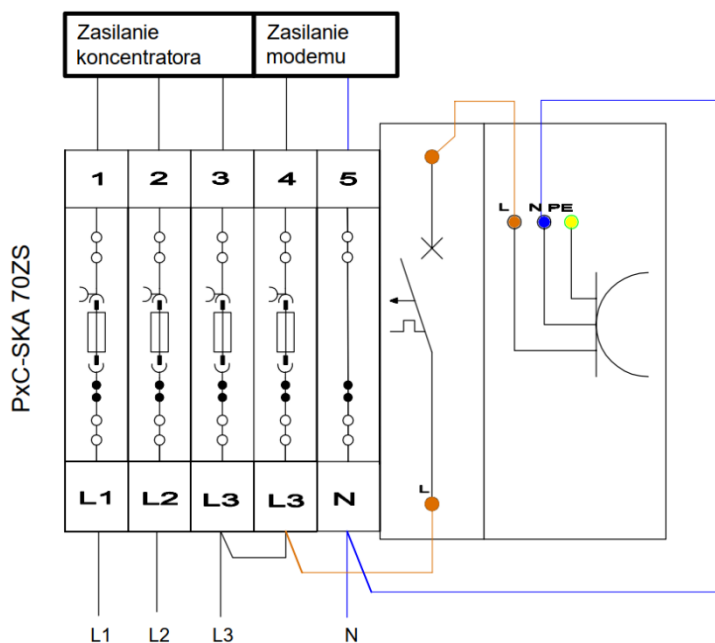
Schemat wewnętrzny listwy PxC-SKA 70ZS
