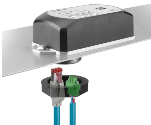
図2：外壁面取り付け図 (FL WLAN 1120)
