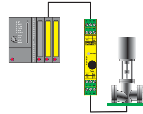
セーフティ PLC の安全出力とフィールドのバルブとを電氣的に絶縁した接続例
