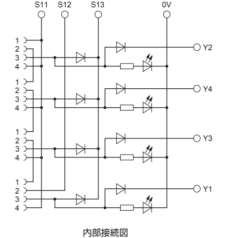
内部接続図
