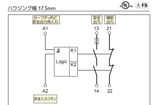
セーフティ PLC の安全出力とフィールドのバルブとを電氣的に絶縁した接続例
