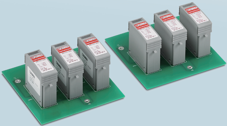
板载式电涌保护器 PRT 系列产品
