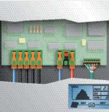
用于逆变器 PCB 板的连接技术
