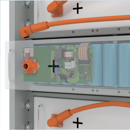
储能电池模块系统插拔式连接器 可实现安全、可靠、灵活的连接。
