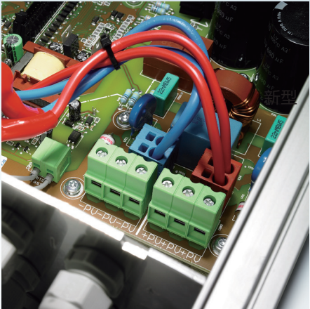
大电流连接器 MKDS 系列
