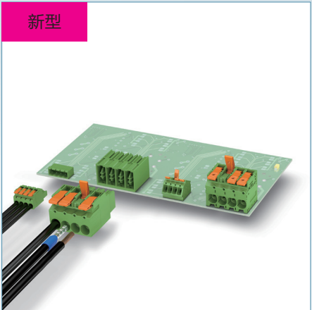
LPT 系列固定式连接器
