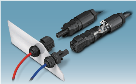
SUNCLIX DC 插拔式连接器 采用弹簧技术,适用于现场布线 (UL 认证)
