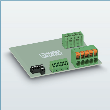
SPT (A) 直插式弹簧系列连接器 TDPT 系列弹簧螺钉兼容连接器
