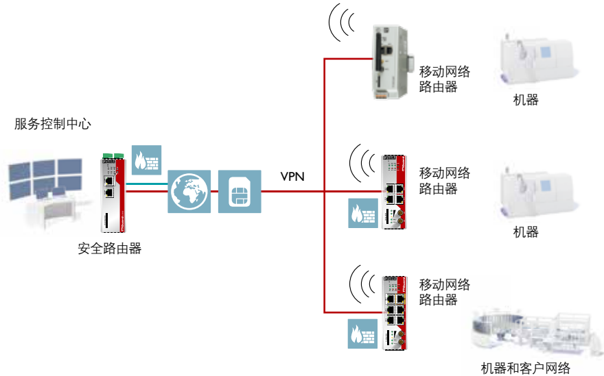
通过移动网络实现VPN通讯
