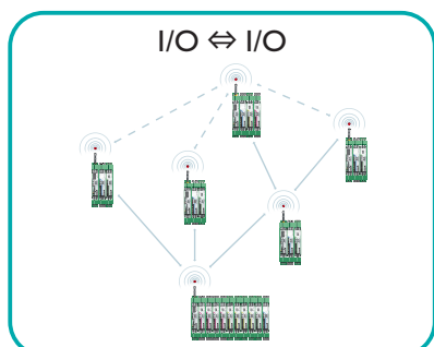
I/O信号伝送と複製。サムホイール操作による簡単な入出力のマッピング
