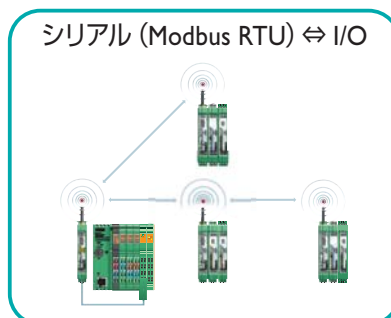
無線経由でデジタル、アナログI/OをMODBUS (RTU) マスタからアクセス可能
