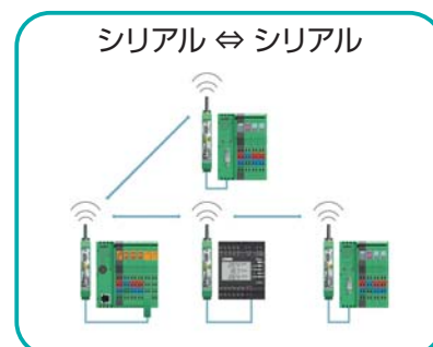
RS232やRS485ケーブルの置き換えにより、MODBUSやPROFIBUSなど様々なプロトコルを透過的に転送
