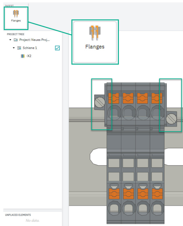
Рис. 9 Фланцы
